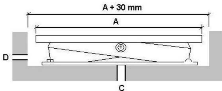
D : TUBE DE MONTAGE, \varnothing = 50 mm D : TUBE \varnothing = 50 mm
