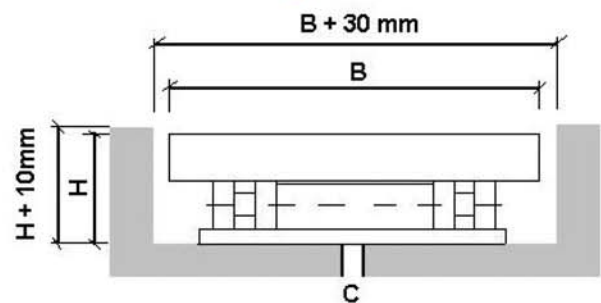
C : TUYAU D'ÉCOULEMENT, \varnothing = 50-100 mm C : OUTLET, \varnothing = 50-100 mm
